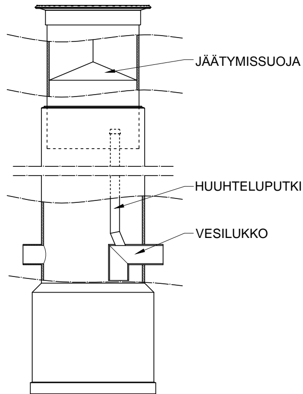
SVK 560/500/170 mittatilauskaivo
